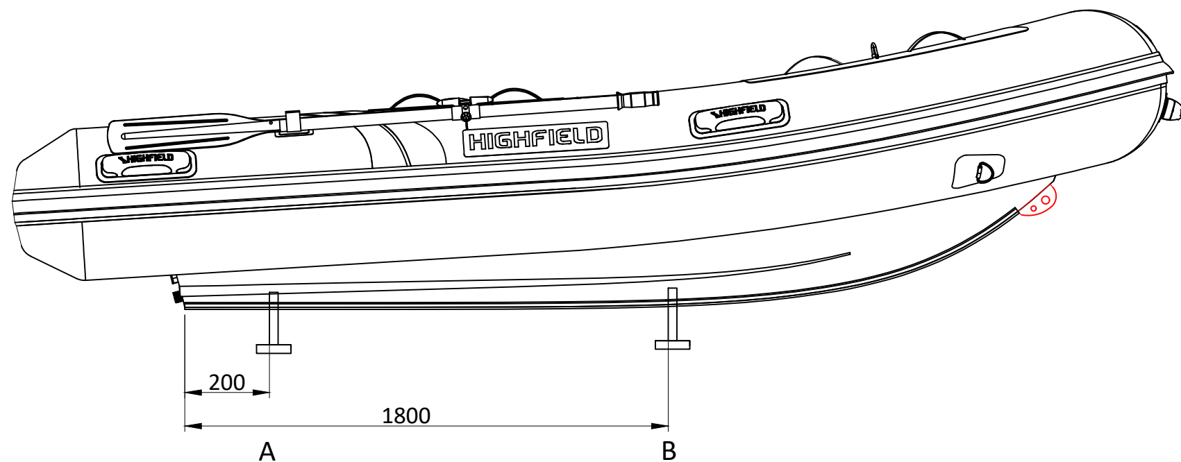
LONGITUDINAL PROFILE
