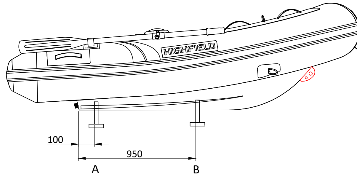
LONGITUDINAL PROFILE
