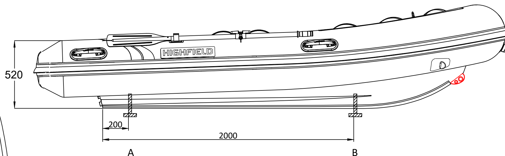
LONGITUDINAL PROFILE
