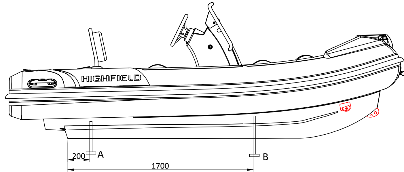
LONGITUDINAL PROFILE
